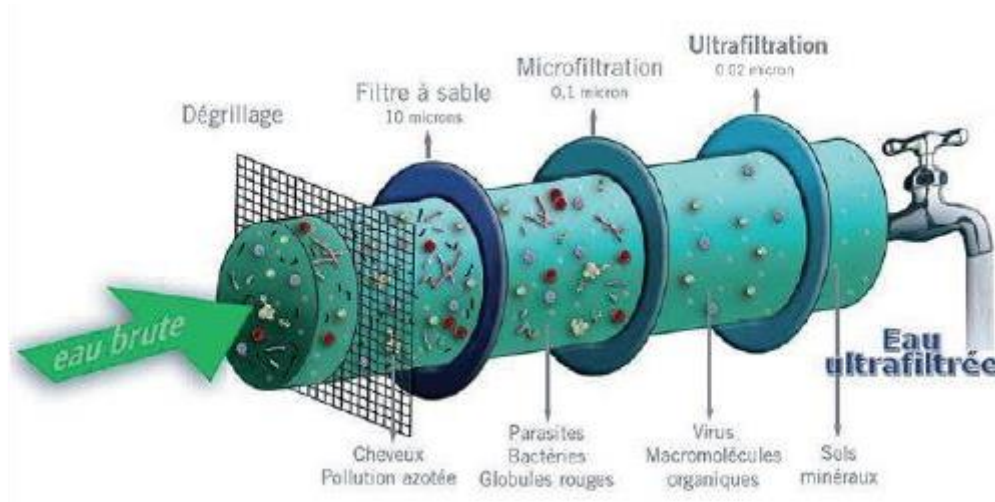
Procédé d'ultrafiltration, retenu pour l'exploitation de la source de Morcueil
