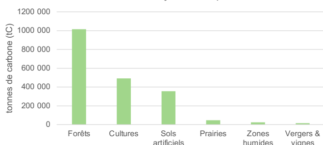
Répartition des stocks de carbone par type de sol - 2018 - Dijon Métropole
