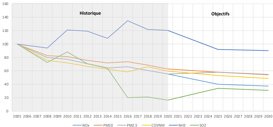
Émissions passées de polluants atmosphériques et objectifs de réduction entre 2005 et 2030 (base 100)
