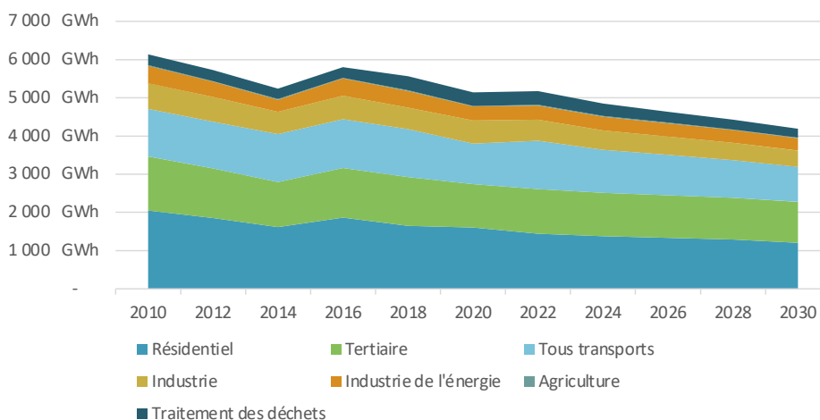
Evolution des consommations énergétiques par secteurs entre 2010 et 2030
